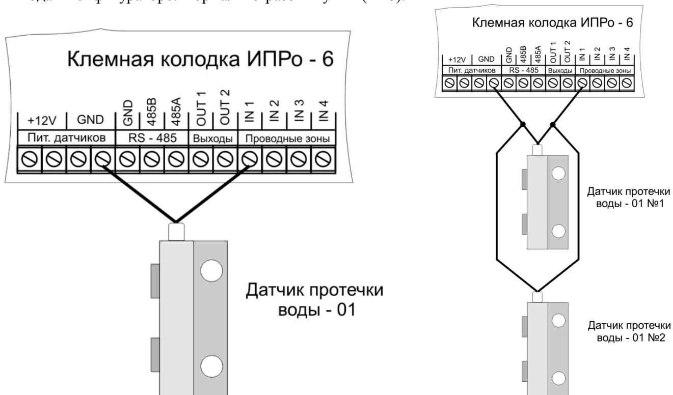
Подключение 1 датчика
