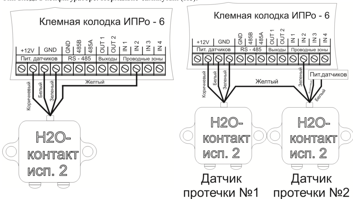
Подключение 1 датчика
